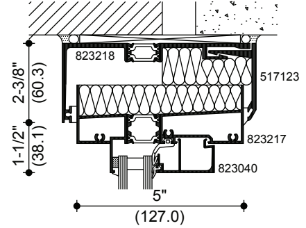
TÊTE ANTIFLEXION (MOUVEMENT ADMISSIBLE DE ± 5/8 PO [15,9 MM])
