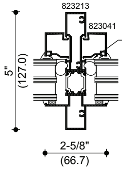
TRIPLE VITRAGE (PEUT LOGER DES UNITÉS SCELLÉES DE 1-3/4 PO [44 MM])
